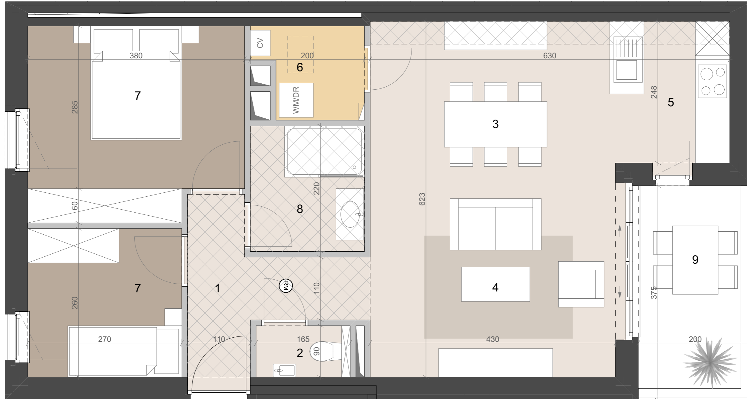
GRONDPLAN
